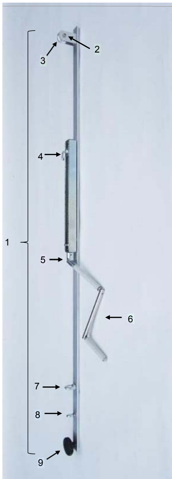
Mechanický napínák
